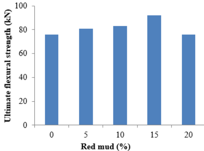
Fig. 7 Flexural strength results [28]
